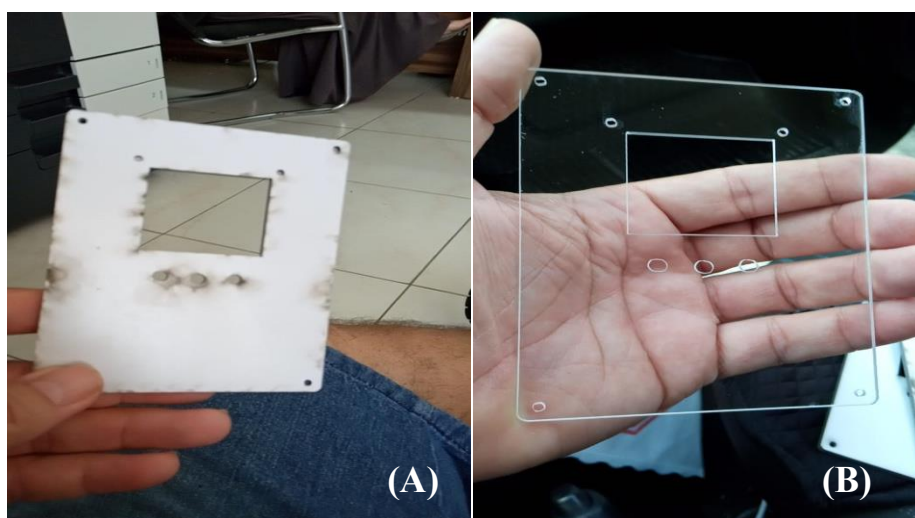
Figura A4 – Corte a laser da placa inicial (A), acabamento final (B).
