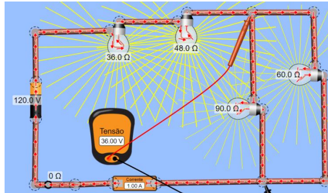
Figura 18: Circuito elétrico com lâmpadas associadas em série e em paralelo, com medida da intensidade de corrente elétrica que passa pela bateria e com a medida da voltagem na lâmpada com resistência de 90\Omega
