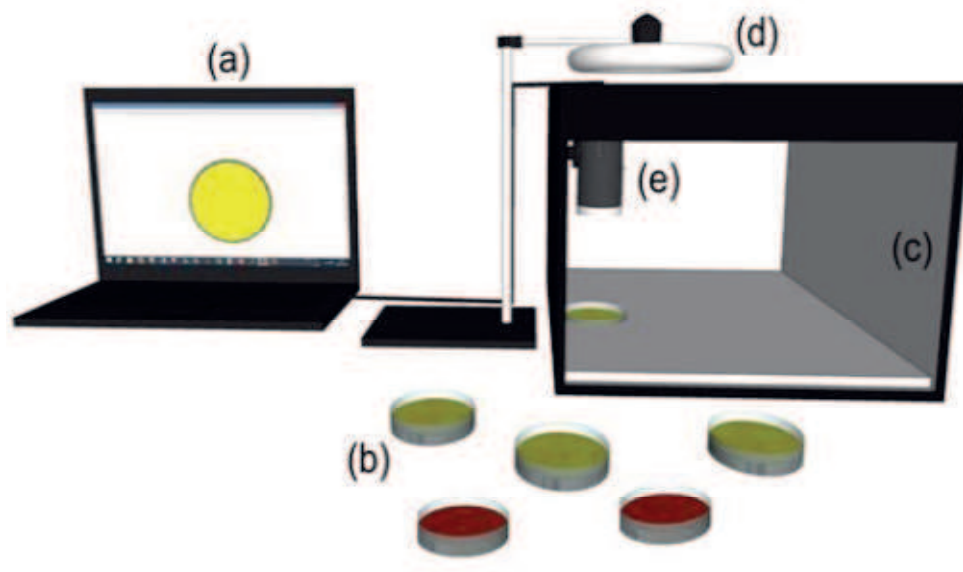
Figure 16 - Sistema utilizado na aquisição das imagens das amostras de biodiesel B100 e B5. (a) notebook; (b) placa de Petri; (c) caixa; (d) lâmpada fluorescente e (e) webcam.
