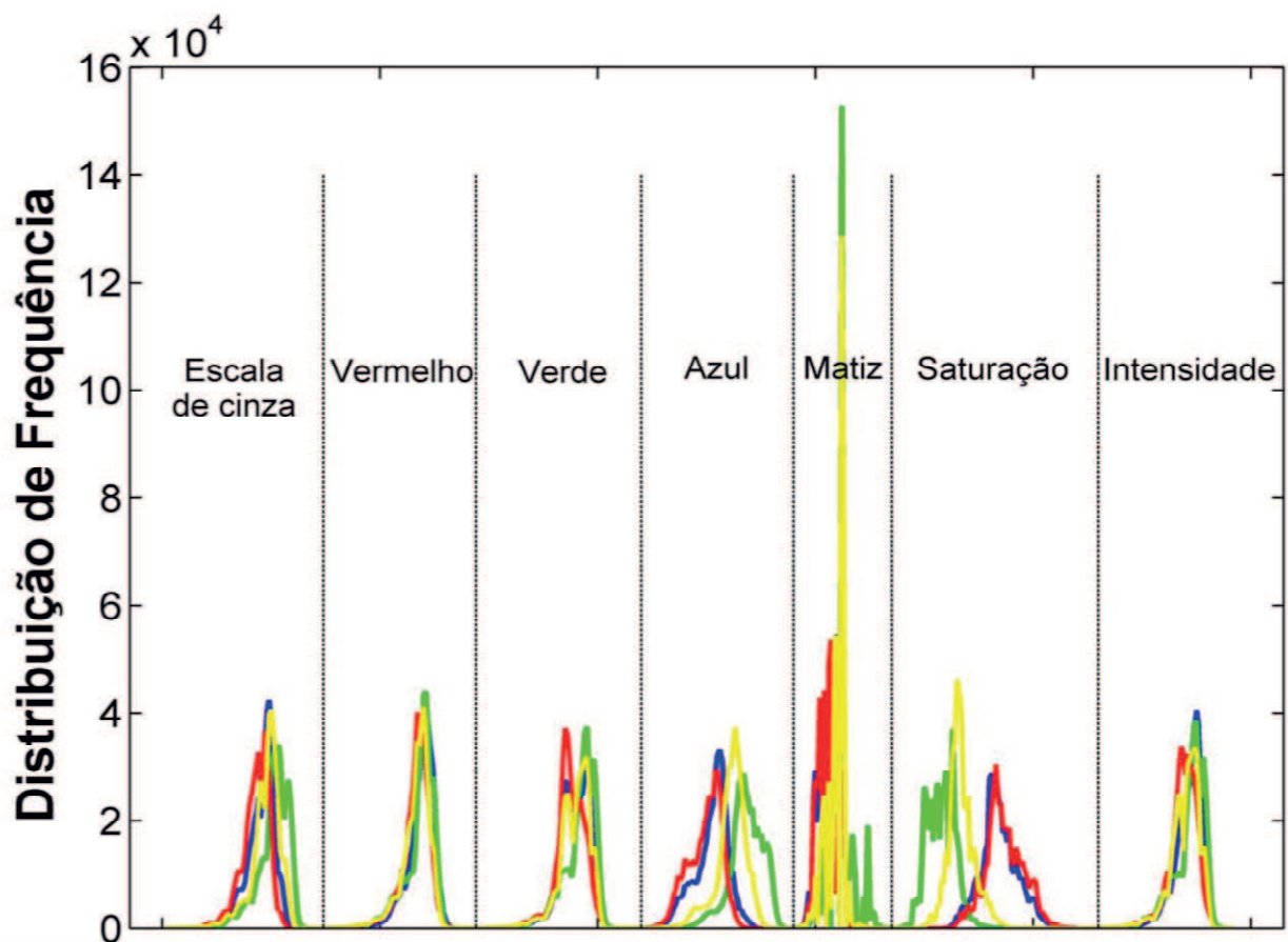
Figure 24 - Histogramas médios nos canais de Escala de Cinza, Vermelho, Verde, Azul, Matiz, Saturação e Intensidade para cada classe de amostras de misturas biodiesel/diesel B5 após a remoção dos zeros: algodão (linha azul), milho (linha vermelha), girassol (linha verde) e soja (linha amarela).
