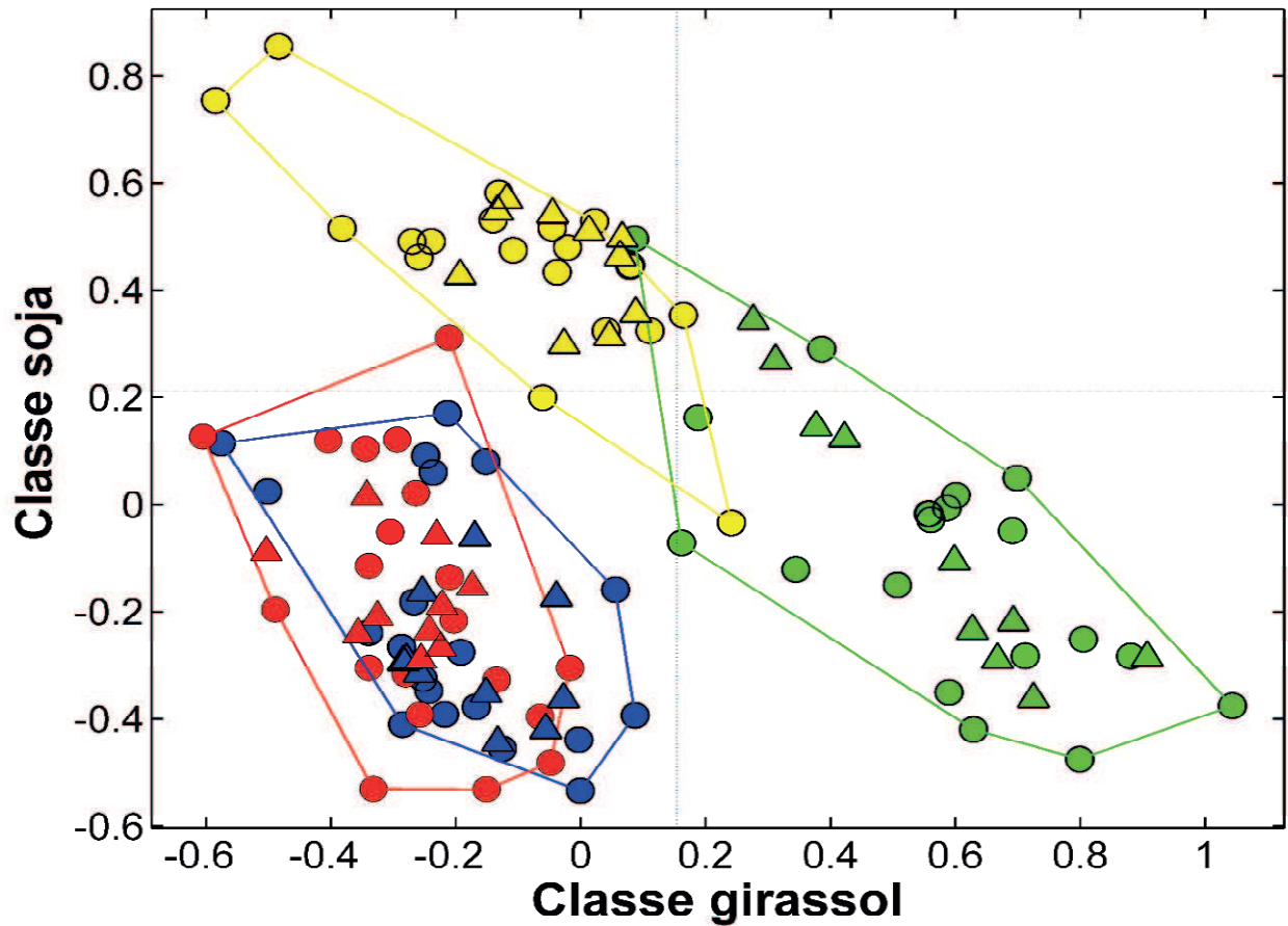
Figura 21 - Gráfico de escores de PLS-DA utilizando o canal Intensidade. Amostras de treinamento (círculo) e teste (triângulo) para os biodiesel B100 de algodão (azul), milho (vermelho), girassol (verde) e soja (amarelo).
