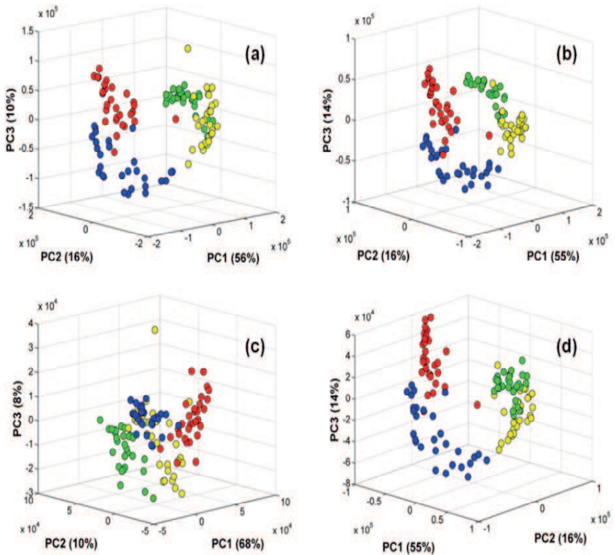
Figura 19 - PCA gráficos dos escores PC1 x PC2, obtidos para as componentes de cores (a) RGB + HSI + Escala de Cinza (b) RGB e (c) Escala de Cinza + HSI para as quatro classes das amostras de biodiesel B100: (●) algodão (●) girassol, (●) milho, (●) soja.
