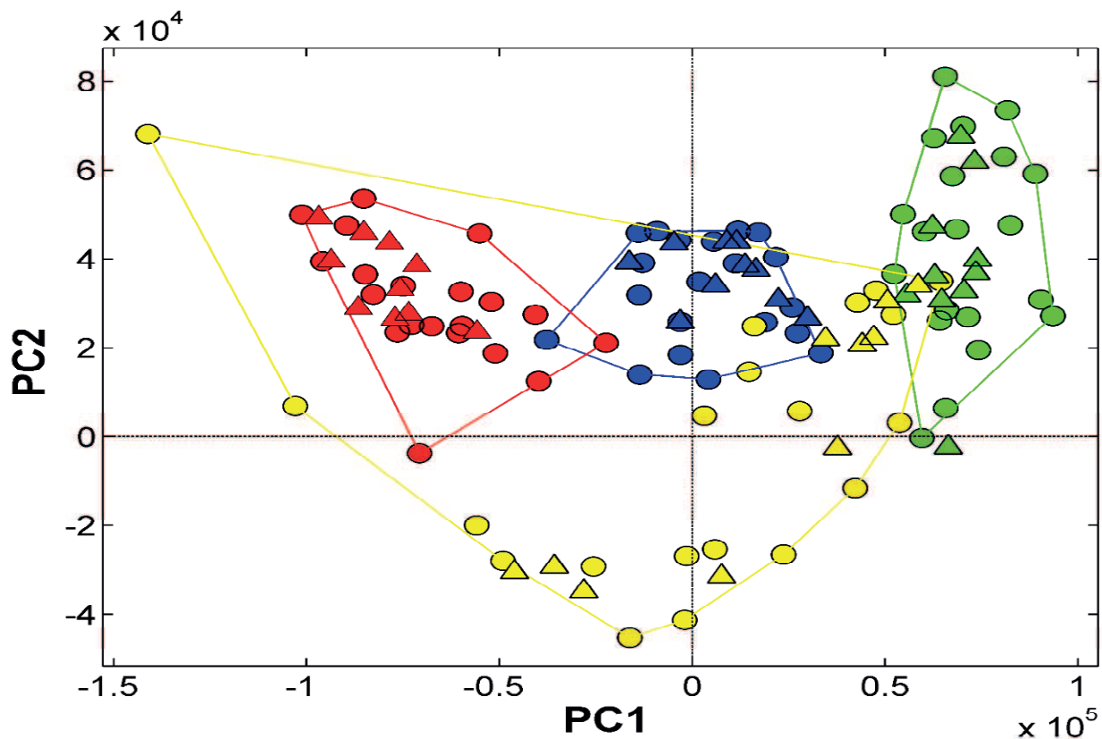
Figura 20 - Gráfico de escores de PC1 x PC2 de SIMCA em relação à classe de soja. Amostras de treinamento (círculo) e teste (triângulo) para os biodieseis B100 de algodão (azul), milho (vermelho), girassol (verde) e soja (amarelo).
