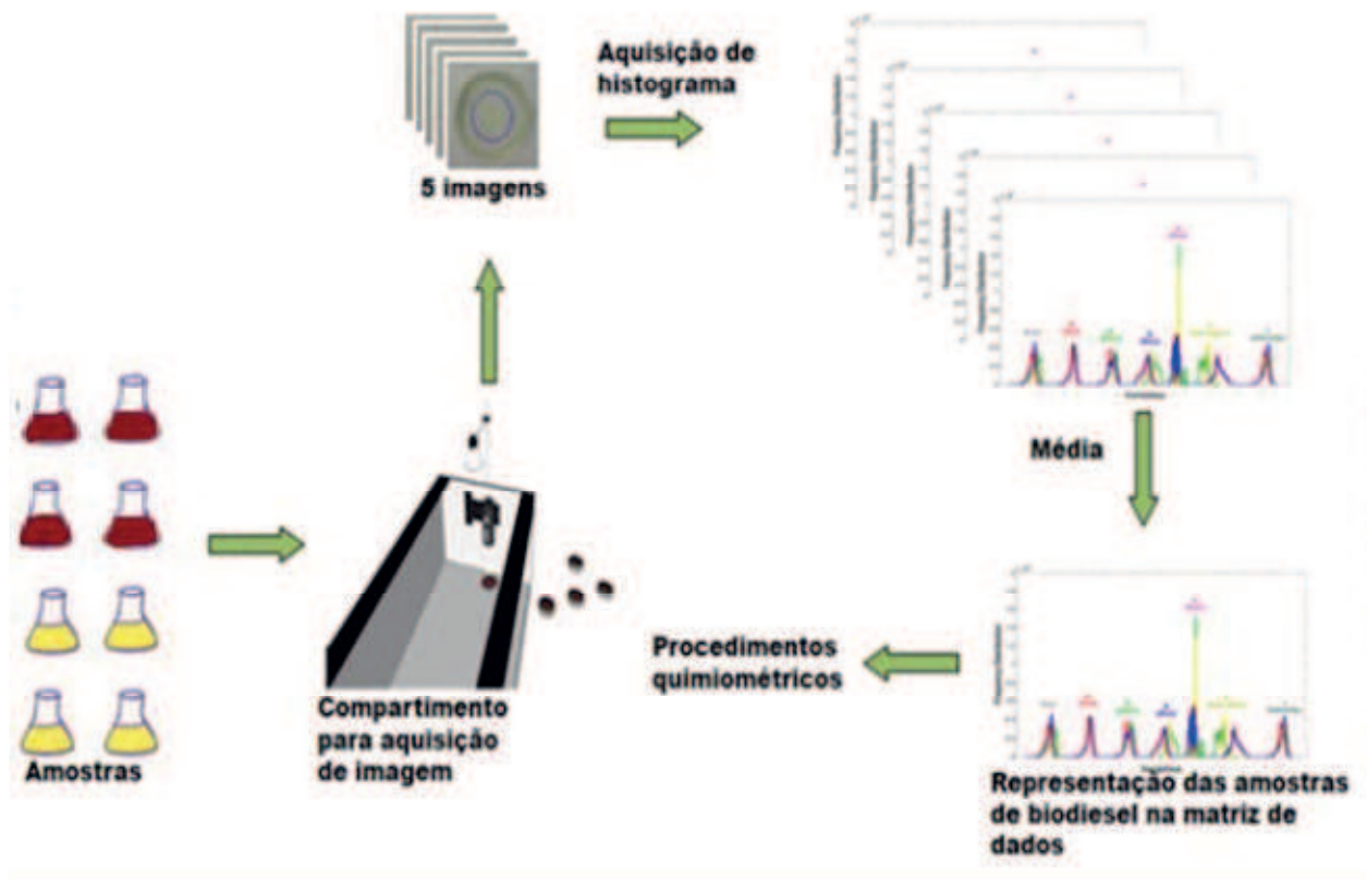
Figura 17 - Representação de amostras na matriz de dados.
