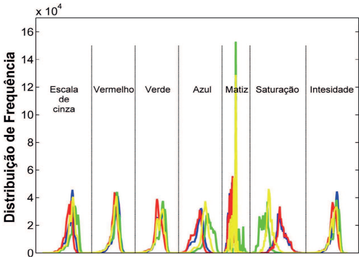
Figura 18 - Histogramas médios nos canais de Escala de Cinza, Vermelho, Verde, Azul, Matiz, Saturação e Intesidade para cada classe de amostra biodiesel B100: algodão (linha azul), milho (linha vermelha), girassol (linha verde) e soja (linha amarela).
