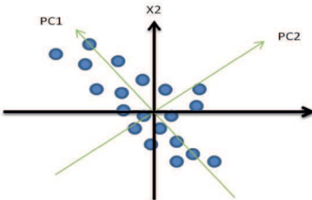
Figura 7 - Posicionamento dos parâmetros da PCA entre duas variáveis originais.
