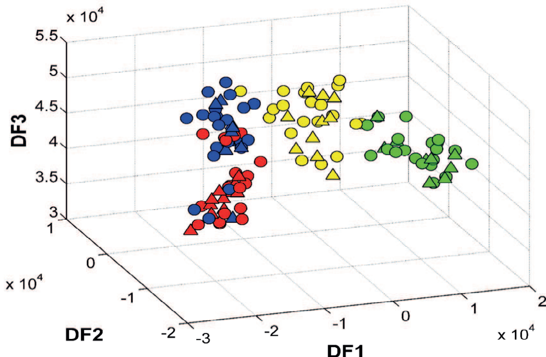
Figura 28 - Funções Discriminantes obtidas pelo SPA-LDA na classificação das 120 amostras de misturas biodiesel/diesel B5: (●) algodão (●) girassol (●) milho, (●) soja.
