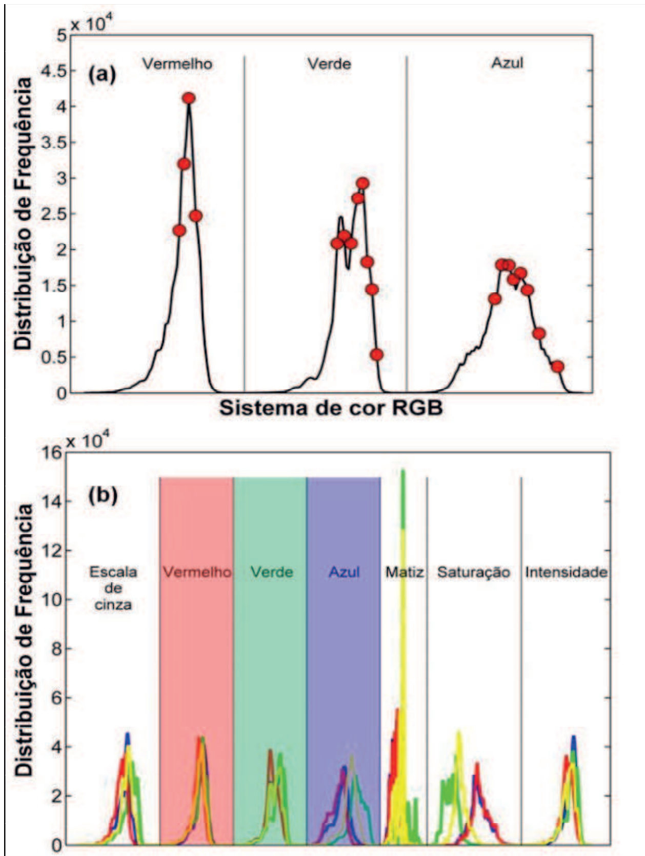
Figura 22 - (a) As 20 variáveis selecionadas pelo SPA para o sistema RGB e (b) distribuição de frequências das cores predominantes para a classificação de amostras de biodiesel B100.
