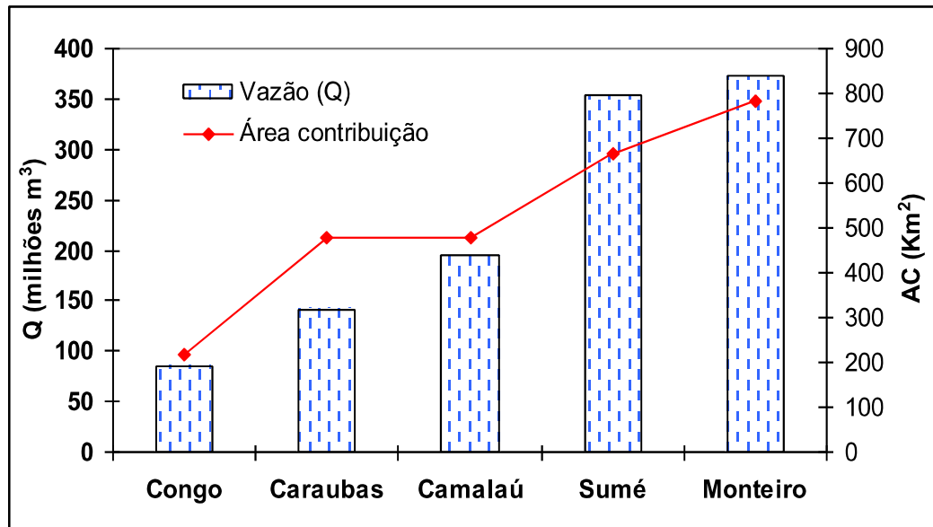
Figura 39. Relação entre a as vazões potenciais- medianas anuais- e as áreas de contribuições da bacia de drenagem do trecho inicial do Alto Curso do rio Paraíba.
